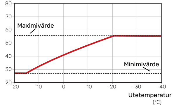
Framledningstemperatur (°C)
