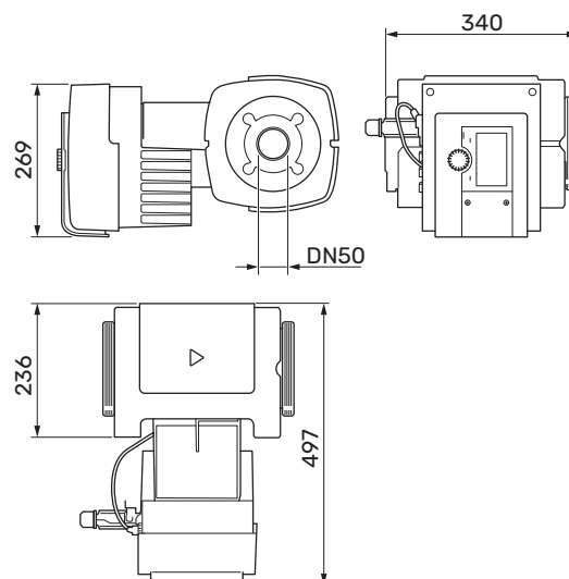
Bipackad köldbärarpump (GP16) 60 kW
