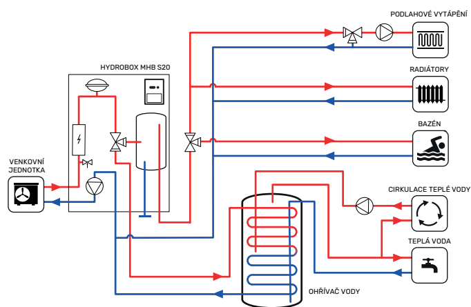
MHB S20 v systému s ohřevem teplé vody, bazénu, okruhu radiátorů a podlahového vytápění se směšováním
