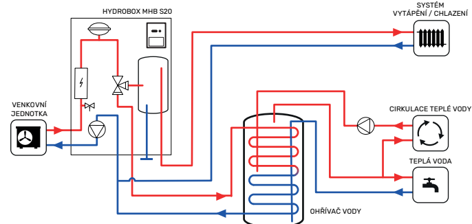
MHB S20 v systému s ohřevem teplé vody a společným okruhem pro vytápění / chlazení
