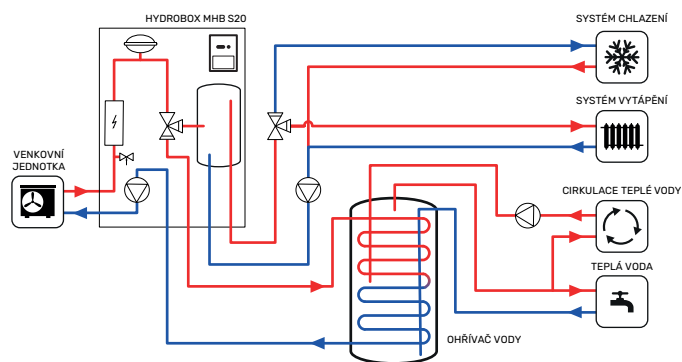
MHB S20 v systému s ohřevem teplé vody a samostatným okruhem pro vytápění / chlazení, vestavěná akumulární nádoba jako oddělovací zásobník
