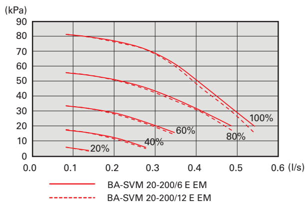
Výtláčny tlak, obehové čerpadlo GP12.
