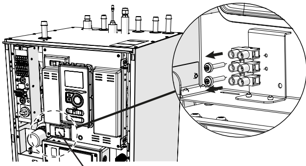
Doska, ktorú je potrebné vyraziť
