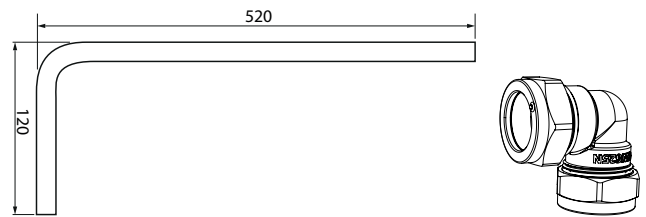
Rozmery cirkulačného potrubia
