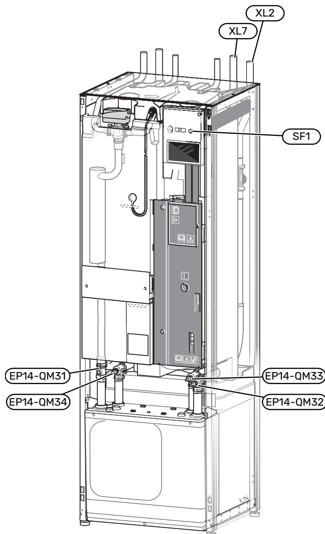
Na obrázku je znázorněn příklad modulu kompresoru.
