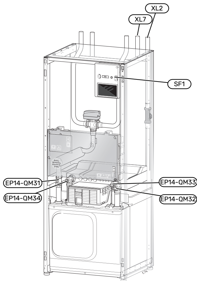
Na obrázku je znázorněn příklad tepelného čerpadla.
