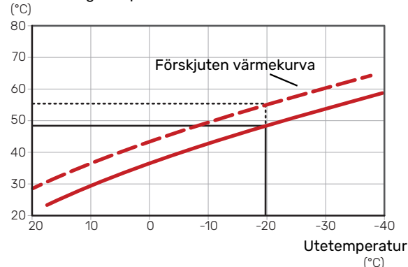
Framledningstemperatur (°C)
