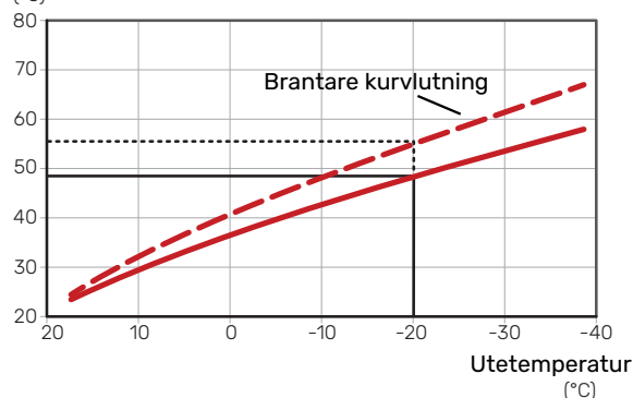
Framledningstemperatur (°C)
