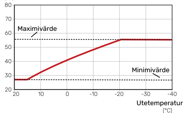
Framledningstemperatur (°C)
