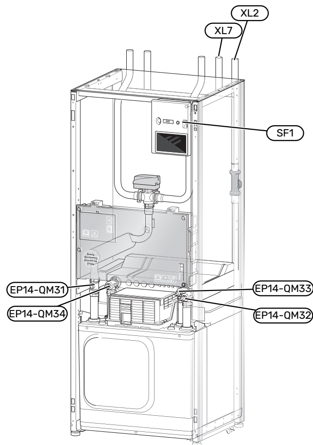
Na obrázku je príklad tepelného čerpadla.
