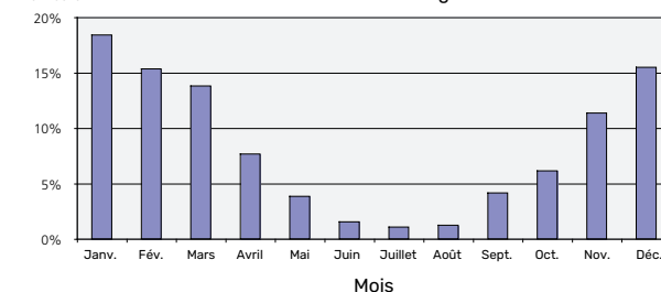
La distribution d'énergie de la pompe à chaleur géothermique s'effectue tout au long de l'année.
