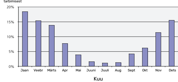
Maasoojuspumba energia jaotus aasta vältel.
