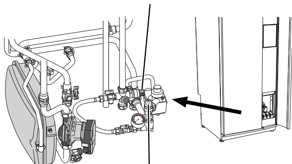
Pojistný ventil pro klimatizační systém
