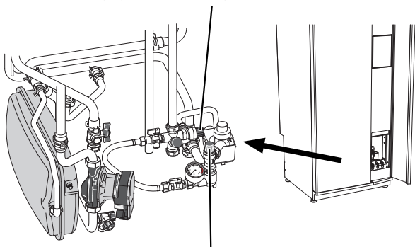
Soupape de sécurité pour réseau de distribution
