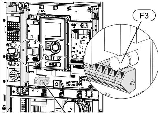
Rikkevoolukaitse RCD
