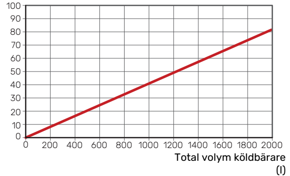
Volym tryckexpansionskärl
