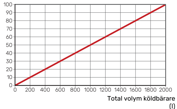
Volym tryckexpansionskärl
