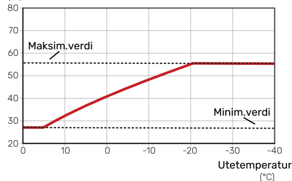
Turledningstemperatur (°C)
