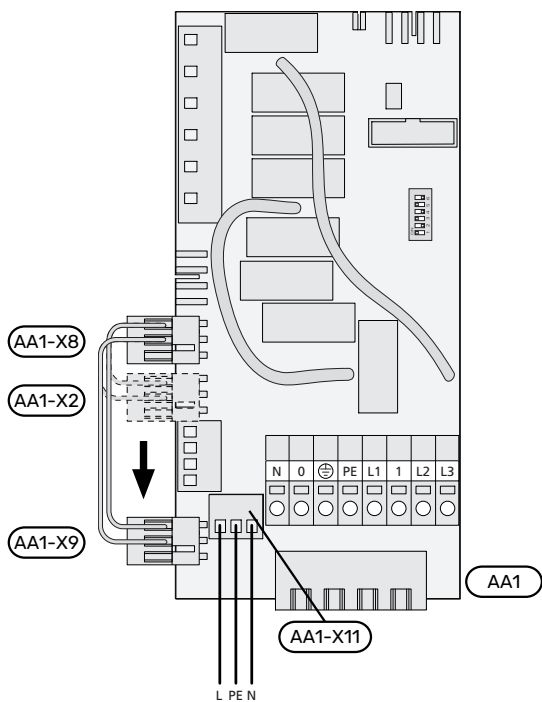
1x230V+N+PE különválasztott villamos megtáplálás
