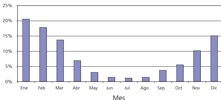
% de consumo anual Consumo de energía de la bomba de calor de aire/agua a lo largo del año
