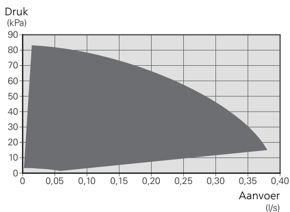
Vermogen, circulatiepomp verwarmingssysteem
