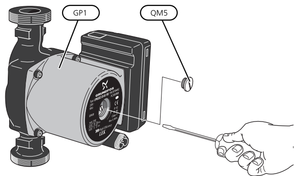
Rysunek przedstawia przykładowy wygląd pompy obieguowej.
