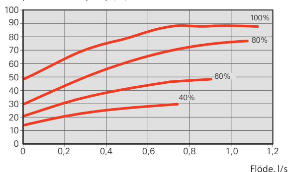
Eleffekt per cirkulationspump (W)
