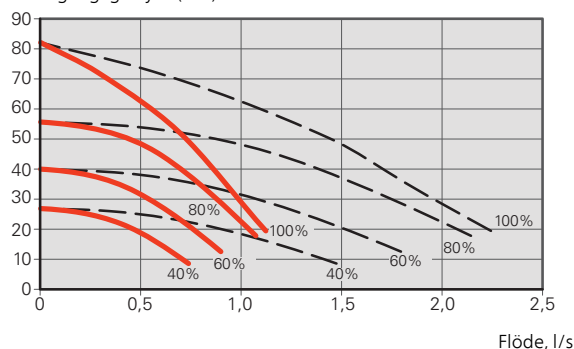
Externt tillgängligt tryck (kPa)
