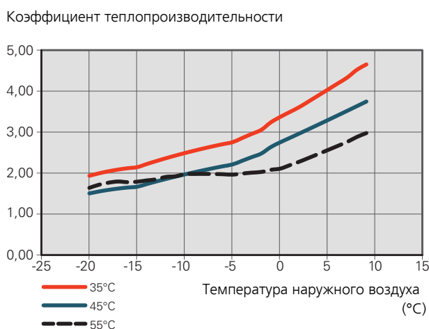
Коэффициент теплопроизводительности F2040-8
