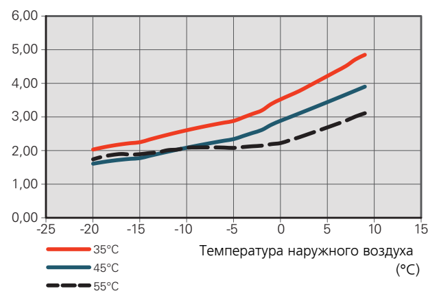
Коэффициент теплопроизводительности F2040-16
