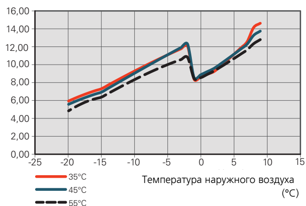
Коэффициент теплопроизводительности F2040-12
