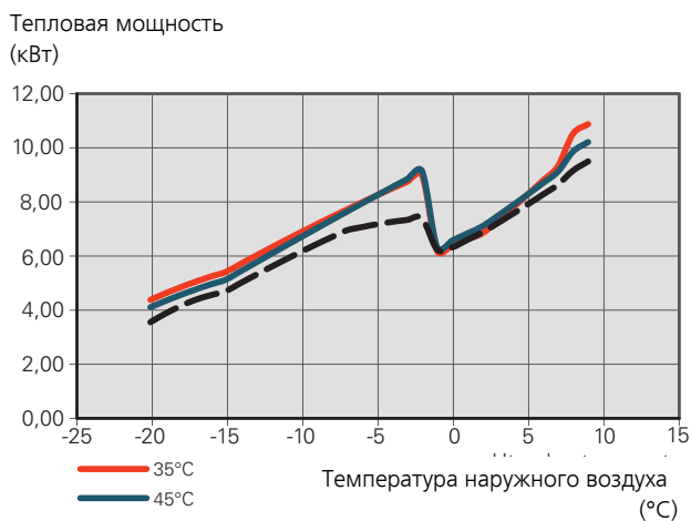
Максимальная заданная выходная мощность F2040-8
