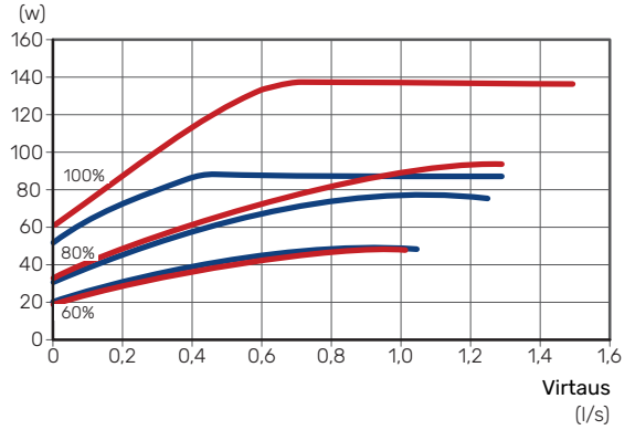
Sähköteho kiertovesipumppu (W)
